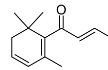
\beta -Damascenon 0,13%
