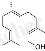
(E,E)-Farnesol
