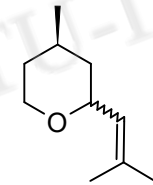
(-) Rosenoxid
