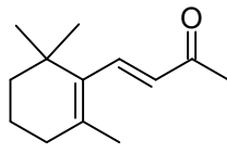
\beta -Ionon 0,03%
